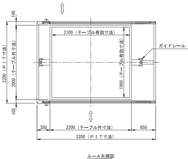
A-A矢視図
